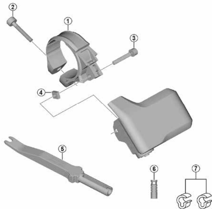
SC-MT800
